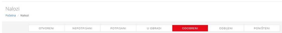
Slika 18 - Statusni izbornik
