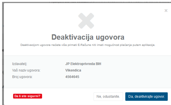
Slika 66. Deaktivacija e-usluge
