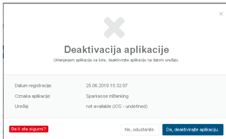
Slika 77. Uklanjanje uređaja
