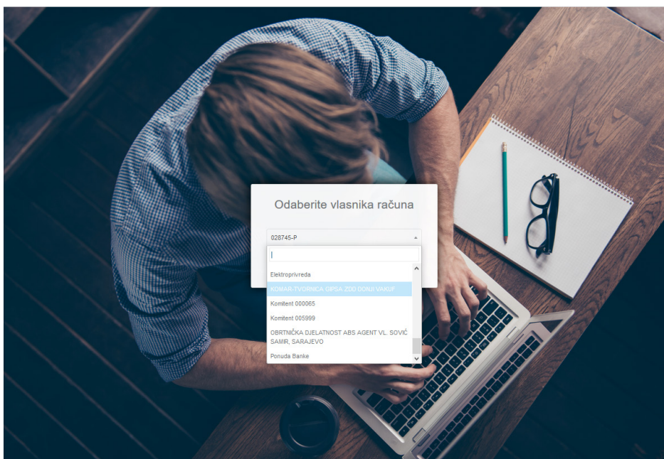
Slika 3 - Odabir vlasnika
