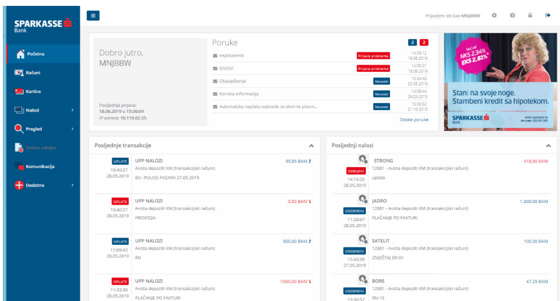
Slika 4 - Početna stranica
