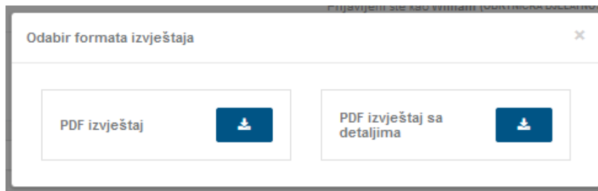
Slika 55. Pregled
