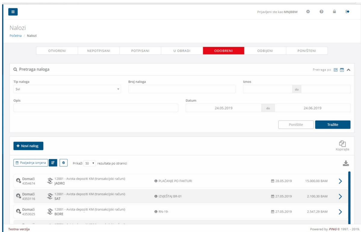
Slika 17 - Modul Nalozi
