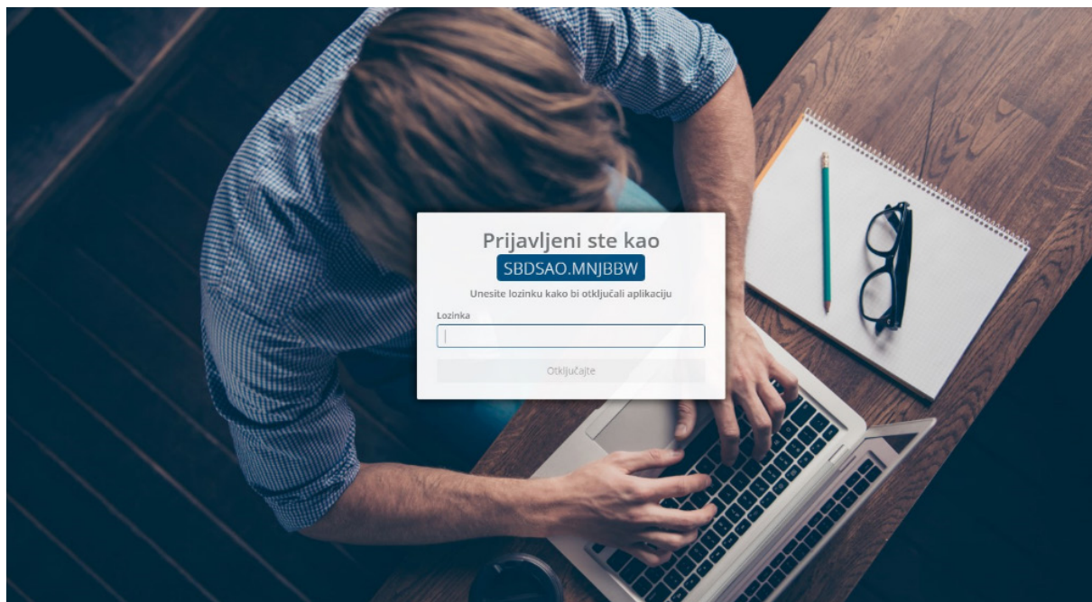
Slika 12 - Zaključavanje aplikacije
